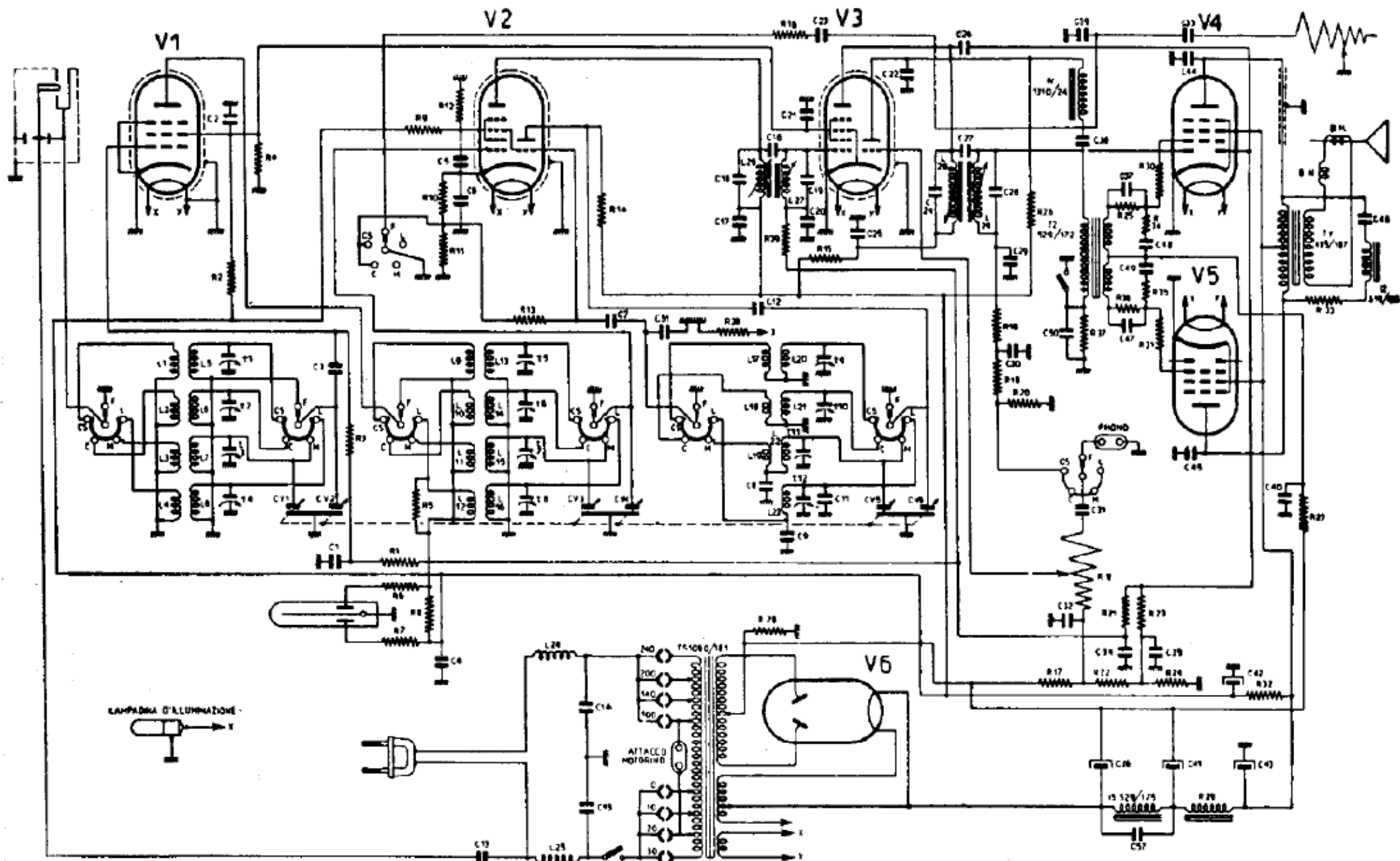
PHONOLA (S. A. FIMI). — Mod. « 622 », — Schema elettrico.
